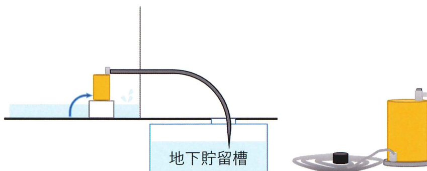
排水・回収用ポンプの準備 (イメージ画像：東京都環境局作成)
