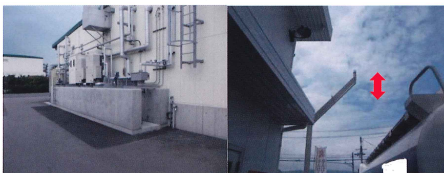
設備等のかさ上げ、通気管のかさ上げの例 （画像出典：危険物施設の風水害対策のあり方に関する検討報告書）
