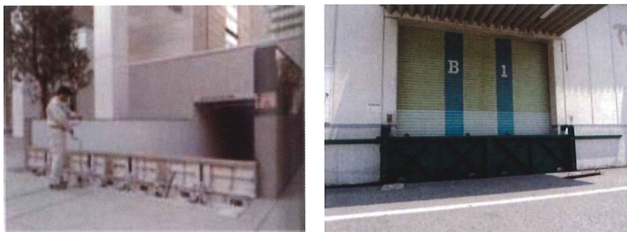
開口部設置型止水板（起立式、スライディング式）の例 （画像出典：危険物施設の風水害対策のあり方に関する検討報告書）
